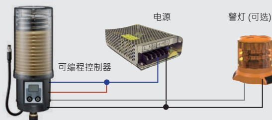
直流配电板接线方法
